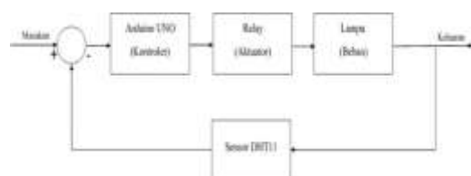
Gambar 3. Blok Diagram Sistem Mesin Penetas Telur
