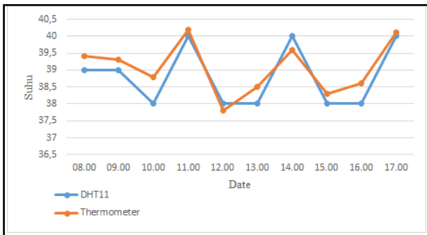
Gambar 9. Grafik Pengambilan Data Suhu Kedua
