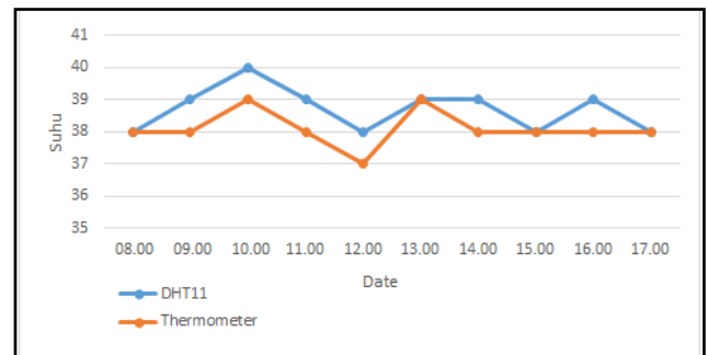
Gambar 7. Grafik Pengambilan Data Suhu Pertama
