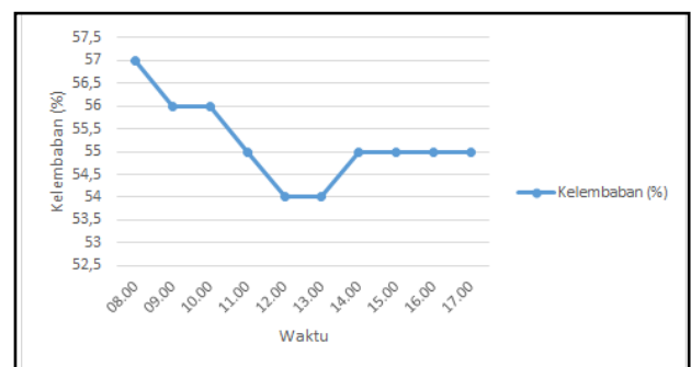
Gambar 8. Grafik Pengambilan Data Kelembaban Pertama
