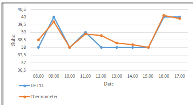
Gambar 11. Grafik Pengambilan Data Suhu Ketiga
