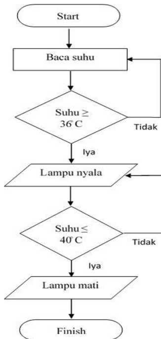
Gambar 4. Flowchart Cara Kerja Mesin Penetas Telur
