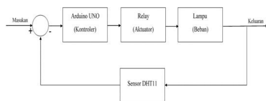
Gambar 3. Blok Diagram Sistem Mesin Penetas Telur
