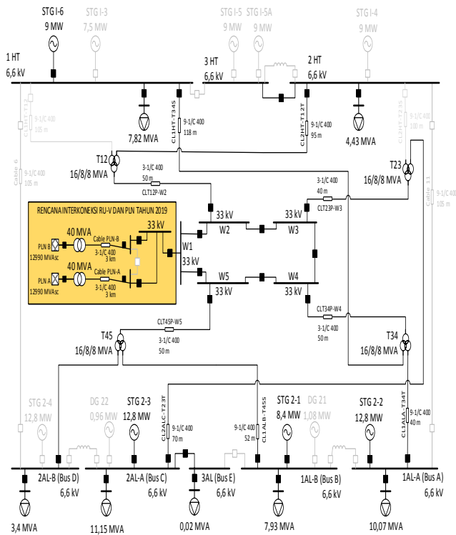
Gambar. 2. Sistem Kelistrikan PT. Pertamina RU V Balikpapan Setelah di Integrasi dengan PLN
