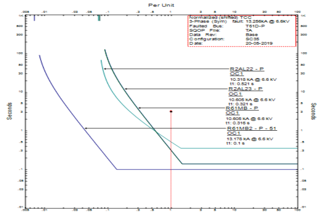
Gambar. 9. Hasil TCC Tipikal 1 ketika Rele 1 Sebagai Pengaman Utama
