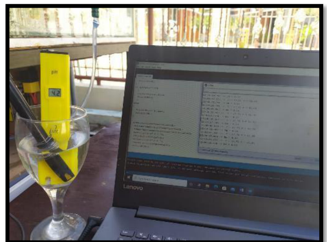
Gambar 4. Kalibrasi Sensor pH dengan pH meter
