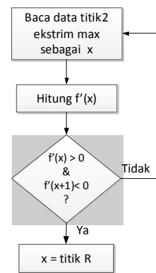
Gambar 4. Algoritma deteksi titik R.
