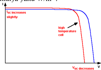
Gambar 1. Efek temperatur pada karakteristik IV sel surya
