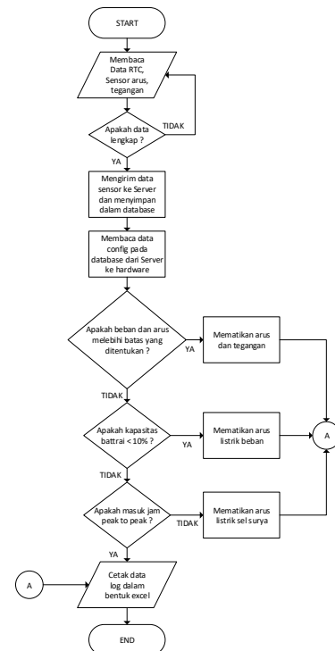
Gambar 4. Flowchart sistem pada perangkat keras
