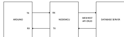
Gambar 3. Komunikasi UART dan WEB API CRUD
