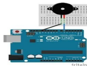
Gambar 4 Arduino dan Buzzer [16]
